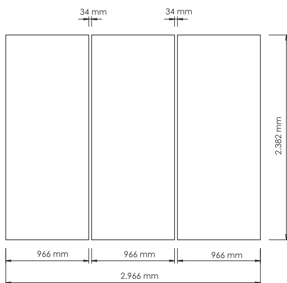
Beispiel einer 3 m Rückwand Example of a 3 m back wall
