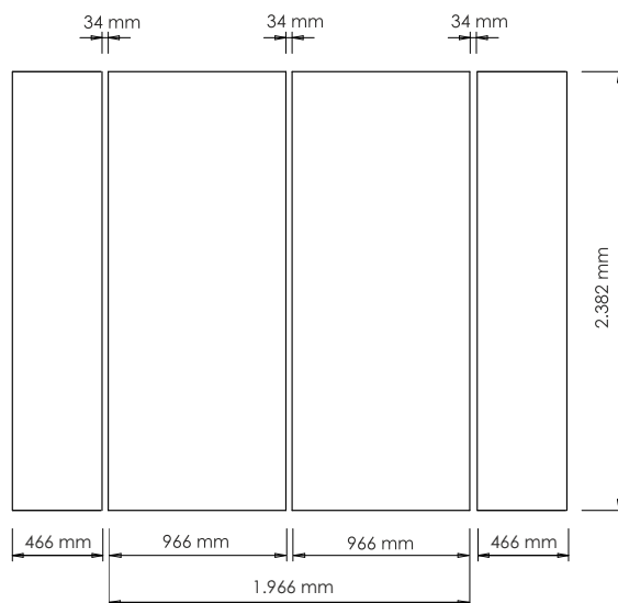
Beispiel einer 2 m Rückwand mit 2 Seitenwänden Example of a 2 m back wall with 2 side walls
